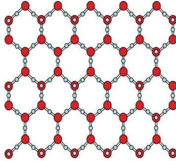
صورة (٣٢): صورة توضح أنّ تنظيم ذرات الماء سداسي.
