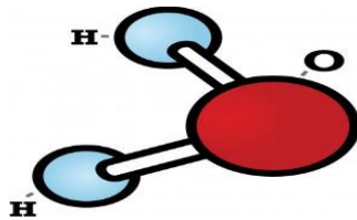
صورة (٣١): جزيئة ماء.
