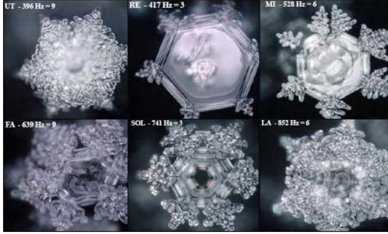
صورة (٣٣): بلورات الماء تترتب على شكل سداسي.
