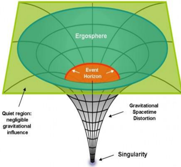
Şekil 22: Kara deliği göstermektedir ve alt kısmında tekillik noktası görünmektedir. 1
