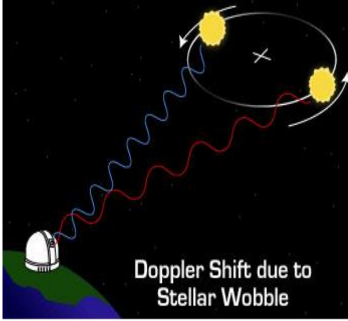
Şekil 26: Doppler olgusunun kullanımına dair başka bir örneğin basitleştirilmiş görseli (Görsel, Doppler farklılığının gezegenleri tespit etmek için nasıl kullanıldığını göstermektedir)
