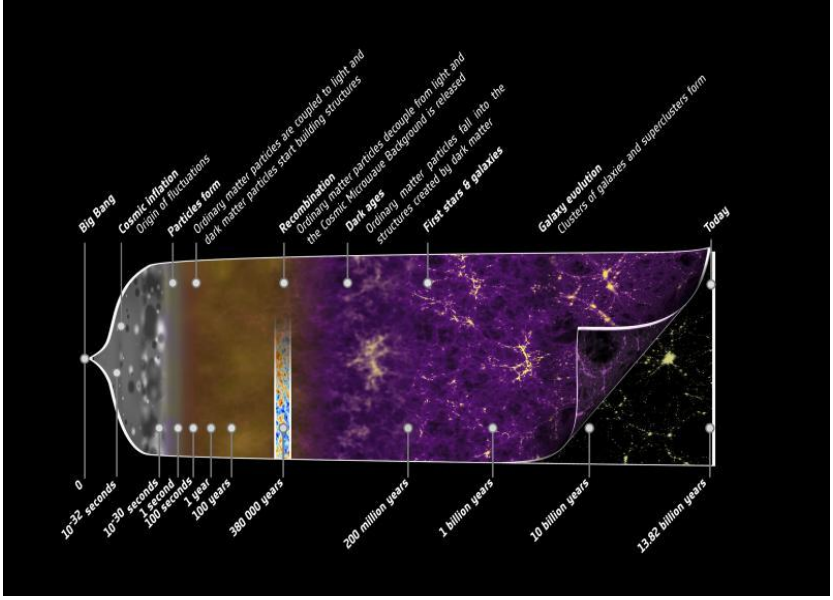
Şekil 29: Büyük Patlama’dan günümüze kadar evrenin oluşum aşamaları 1
