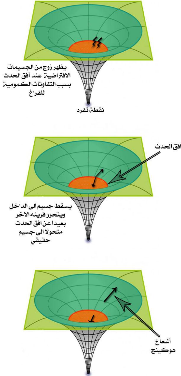
Şekil 23: Hawking ışıının nasıl ve nerede oluştuğunu göstermektedir.
