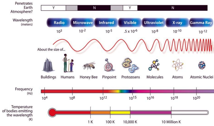
Şekil 21: Elektromanyetik dalgalar, alanları, frekansları ve frekans ile enerji (veya ısı) arasındaki ilişki. Kaynak: NASA Uzay Ajansı.
