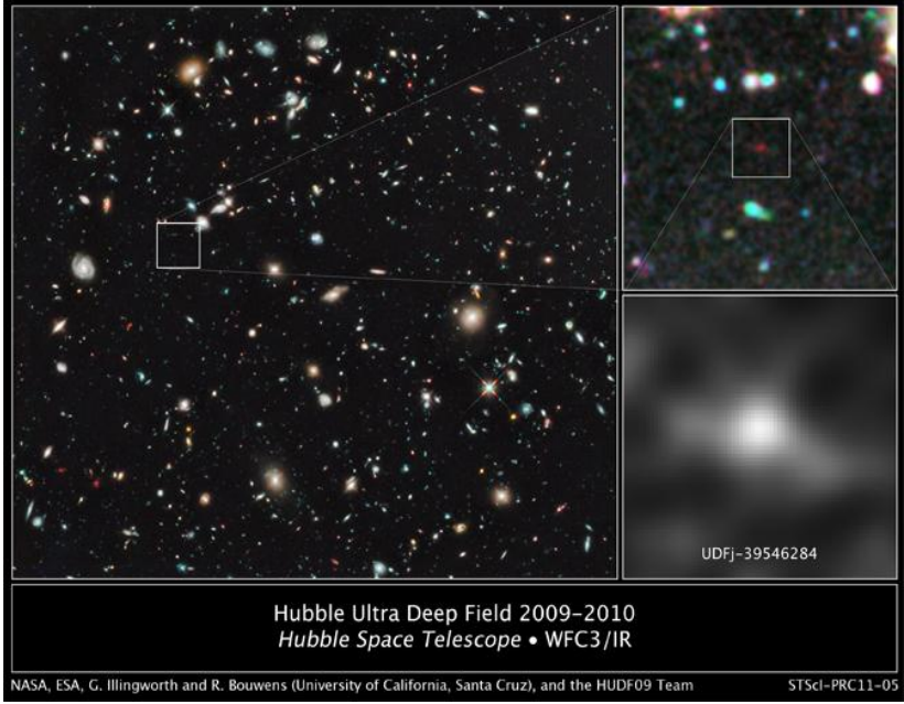
Şekil 28: Renk ölçümüne dayanarak yaklaşık 13,2 milyar ışık yılı uzaklıkta olduğu düşünülen, bilinen en eski galaksilerden birinin görüntüsü. 1
