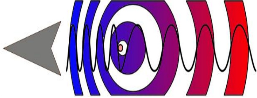
Şekil 25: Doppler etkisinin basit şematik gösterimi 1
