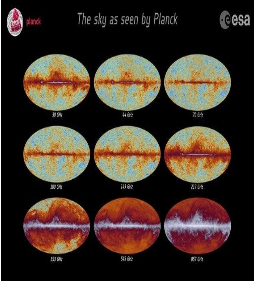
Şekil 27: Planck uzay gözlemevi tarafından farklı frekanslarda çekilmiş gökyüzü haritaları.
